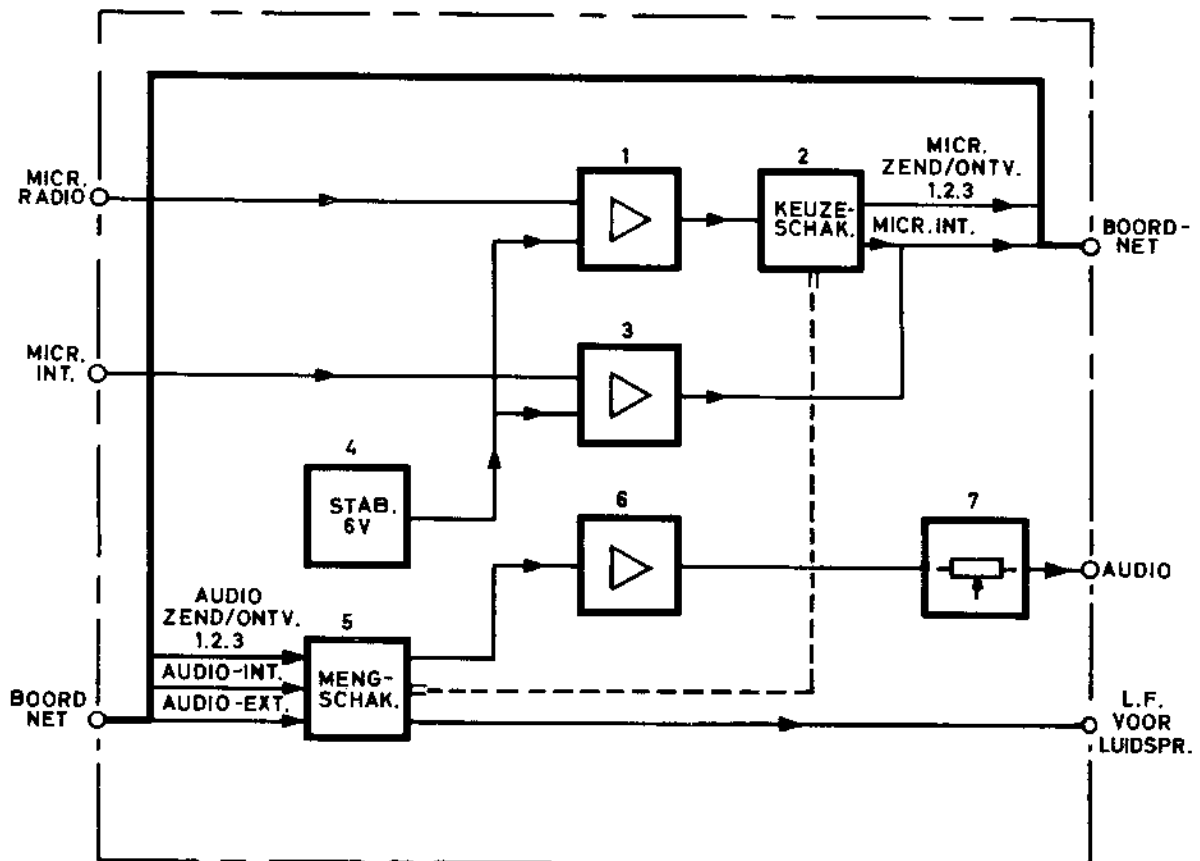
FIGUUR 10 BLOKSCHEMA, SCHAKELKAST C-3621
