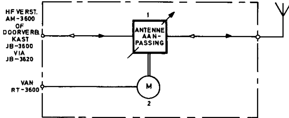
FIGUUR 7 BLOKSCHAMA, ANTENNE-EENHEID RF-3620
