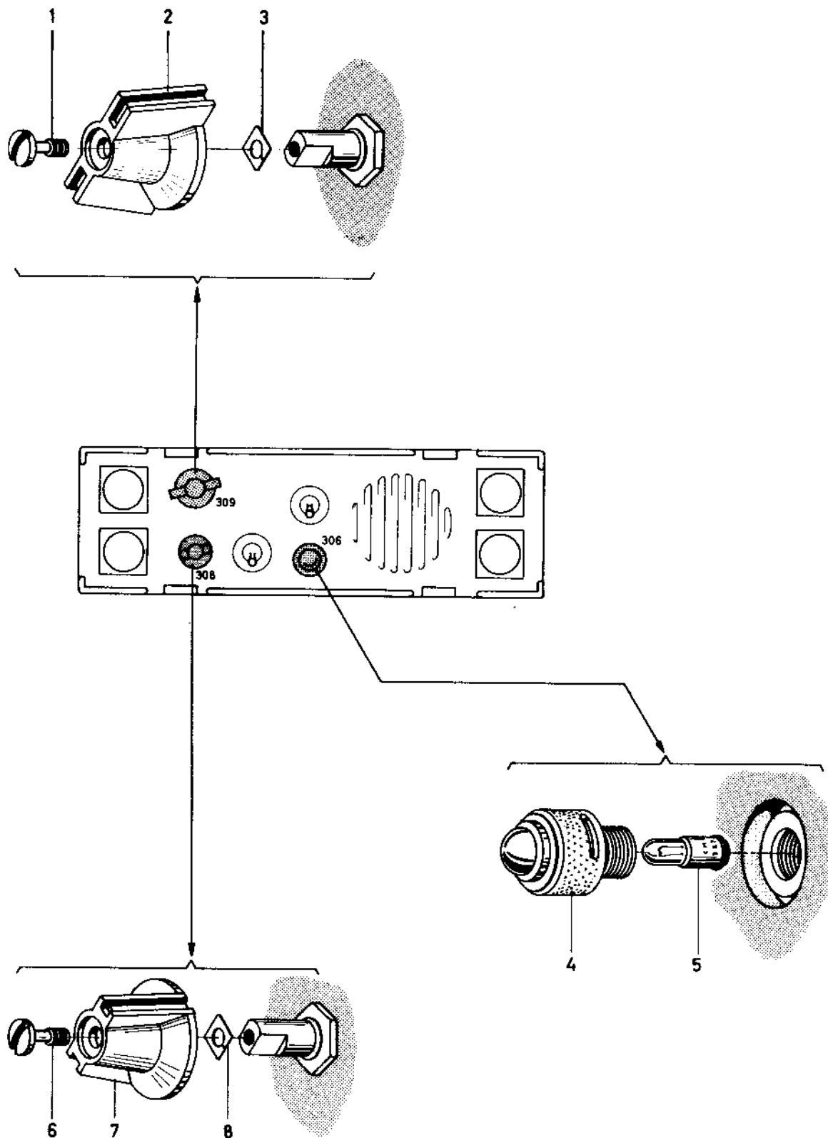
FIGUUR 64 REPARATIE VAN DE REGEL- EN LUIDSPREKEREENHEID AF-3620
