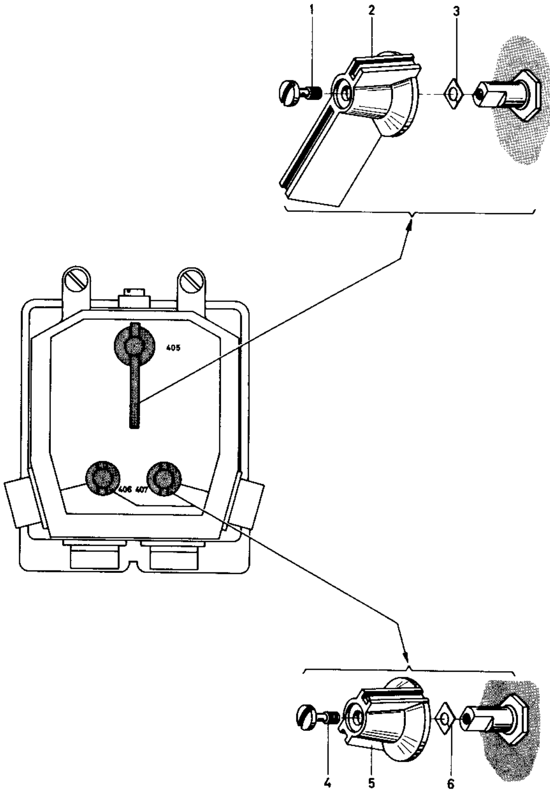
FIGUUR 65 REPARATIE VAN DE SCHAKELKAST C-3621
