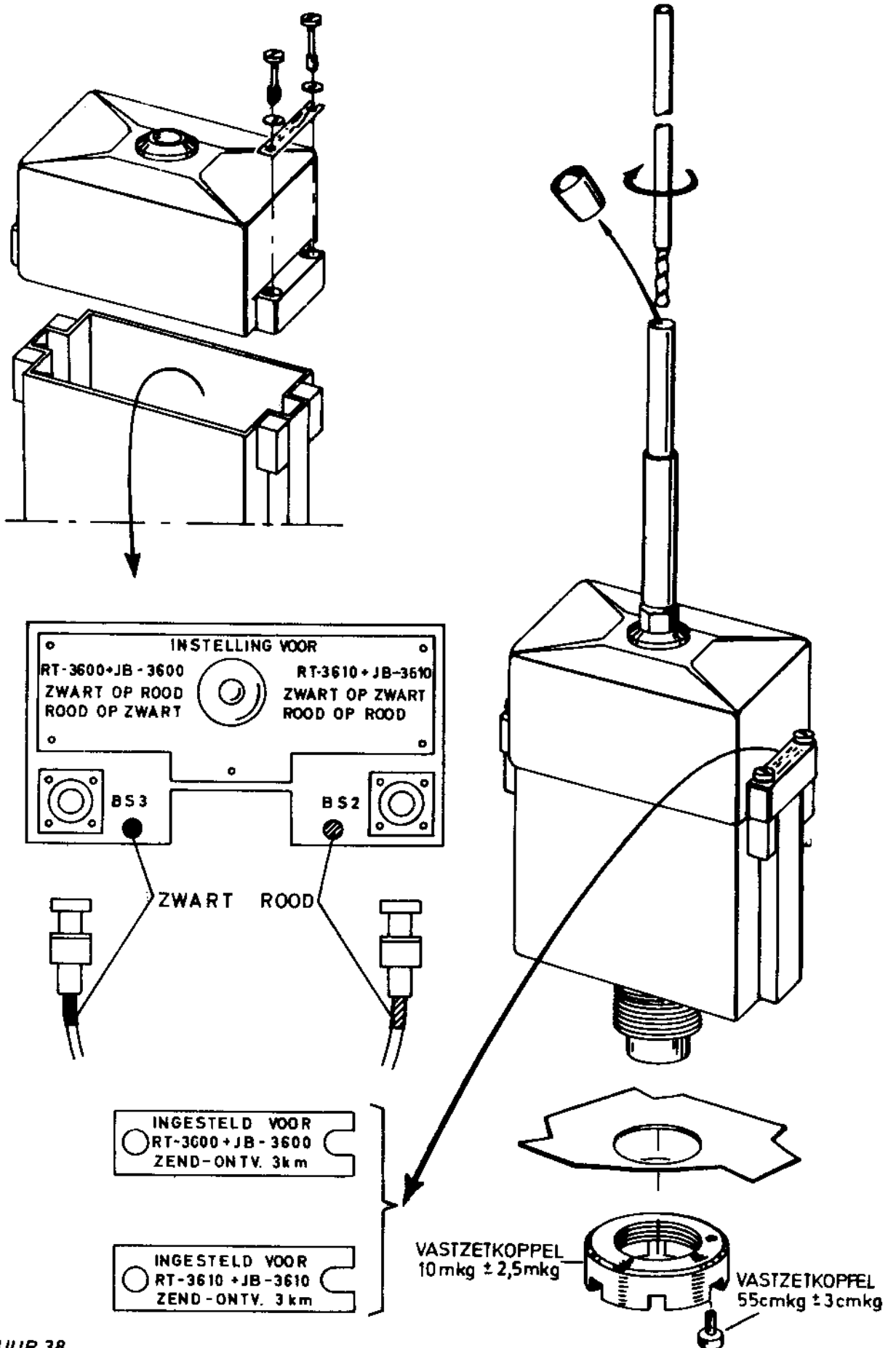
FIGUUR 38 HET INSTALLEREN VAN DE ANTENNE-AFSTEMEENHEID RF-3610
