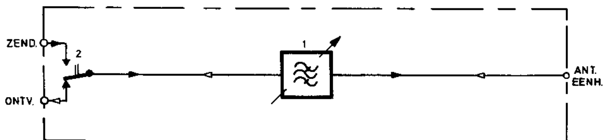
FIGUUR 5 BLOKSCHEMA, DOORVERBINDINGSKAST JB-3600
