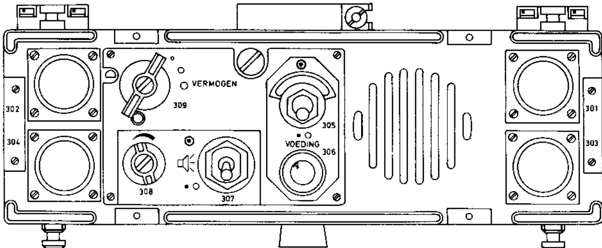
FIGUUR 25 VOORAANZICHT, REGEL-EN LUIDSPREKEREENHEID AF-3620
