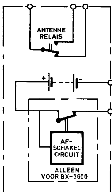
FIGUUR 3 BLOKSCHEMA, BATTERIJHOUDER BX-3600/BX-3601
