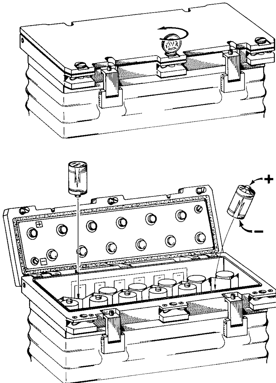
FIGUUR 56a HET VERVERGEN VAN DE BATTERUEN IN DE BATTERIJHOUDER BX-3601
