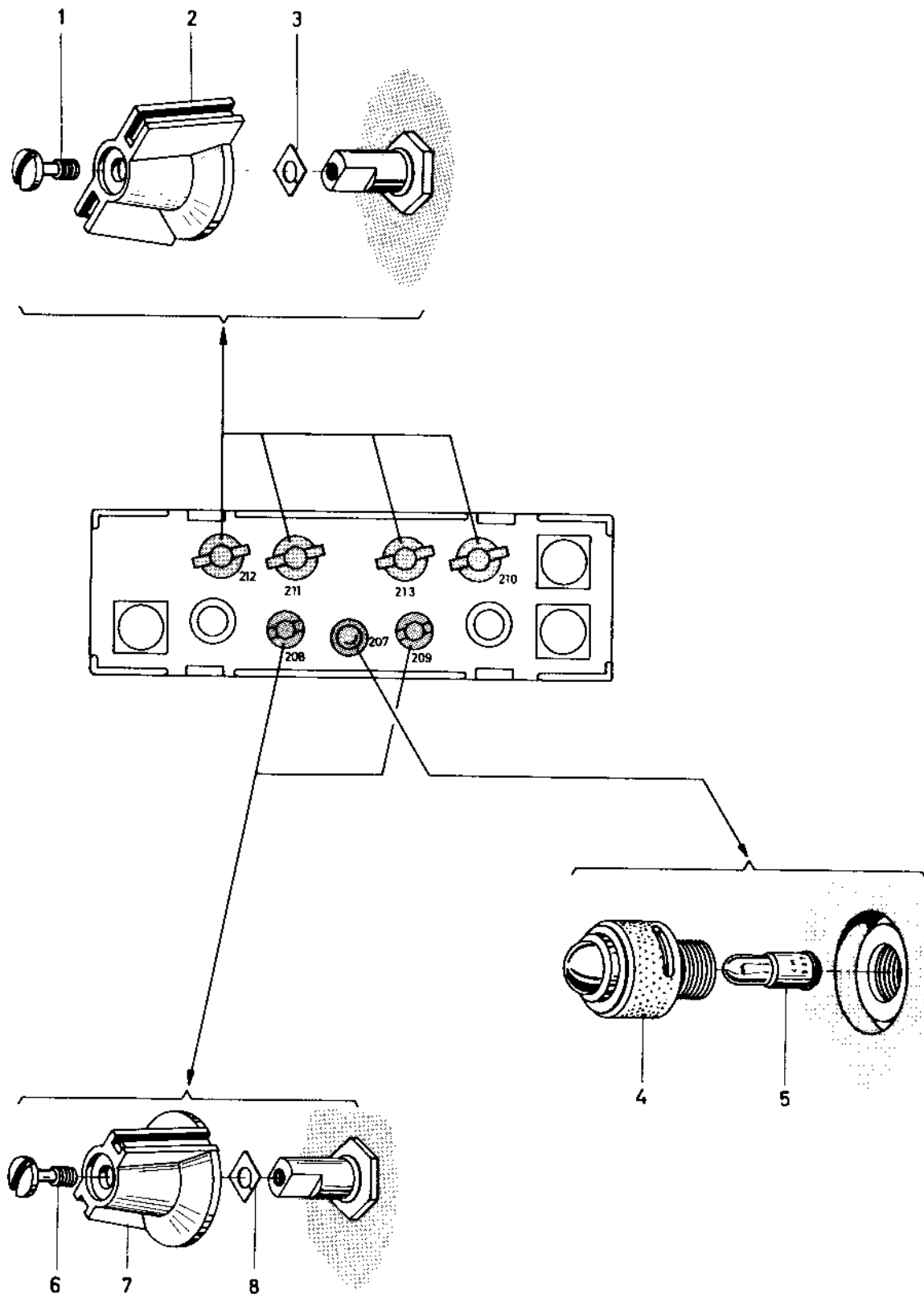
FIGUUR 63 REPARATIE VAN DE REGEL-EN INTERCOMMUNICATIE-EENHEID IC-3620
