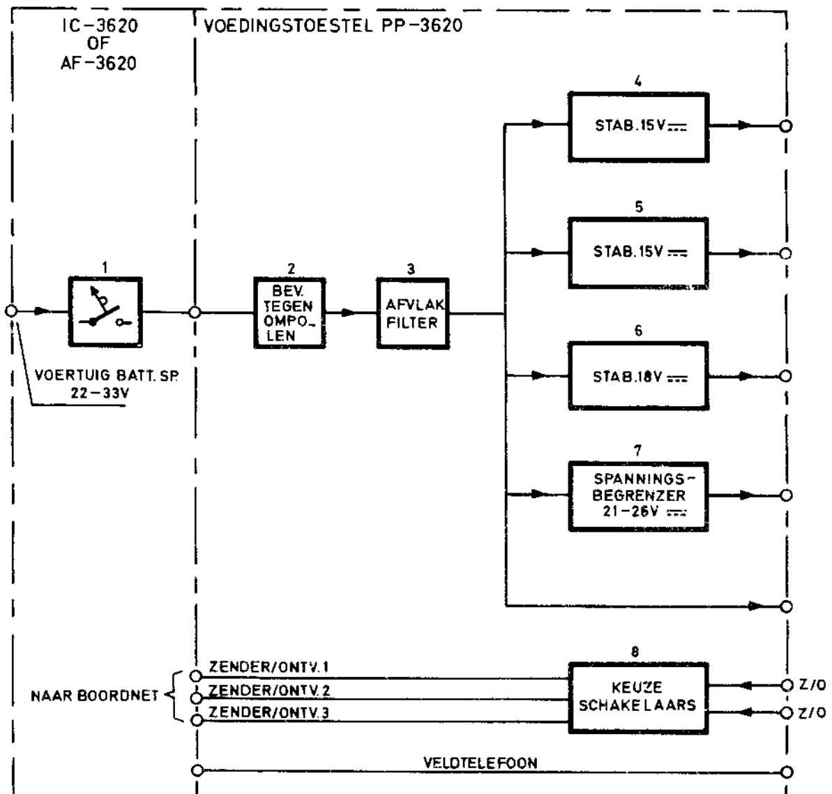
FIGUUR 2 BLOKSCHAMA, VOEDINGSTOESTEL PP-3620
