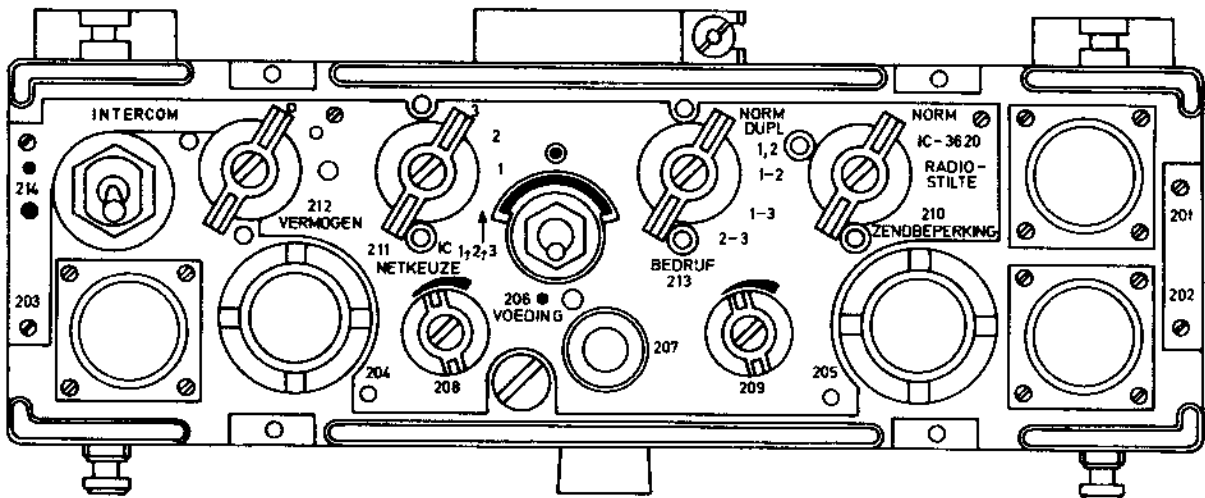
FIGUUR 24 VOCORAANZICHT, REGEL-EN INTERCOMMUNICATIE-EENHEID IC-3620
