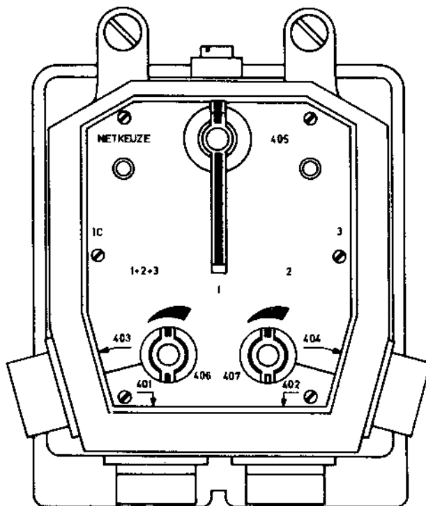
FIGUUR 26 VOORAANZICHT, SCHAKELKAST C-3621
