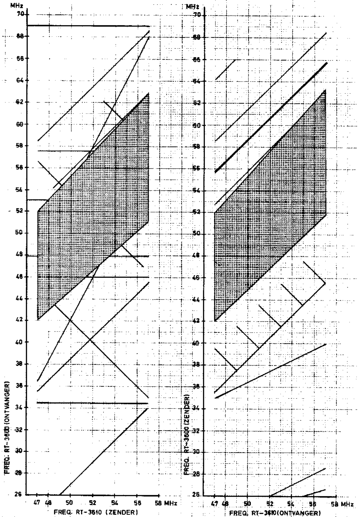
FIGUUR 46 INTERFERENTIEKAART RT-3610/RT-3600
