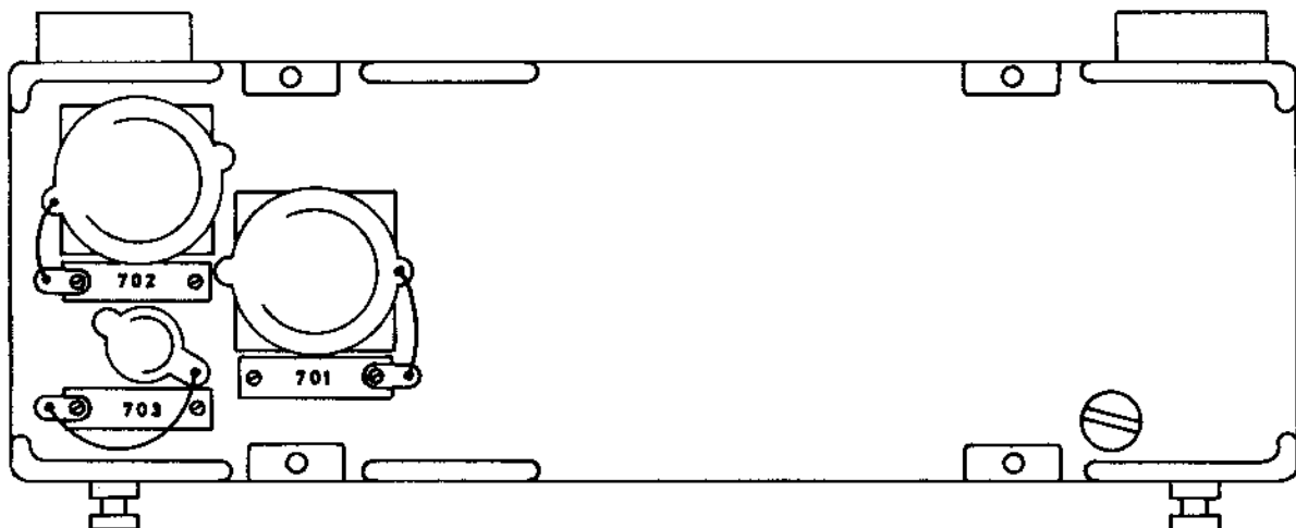
FIGUUR 18 VOORAANZICHT, DOORVERBINDINGSKAST JB-3600
