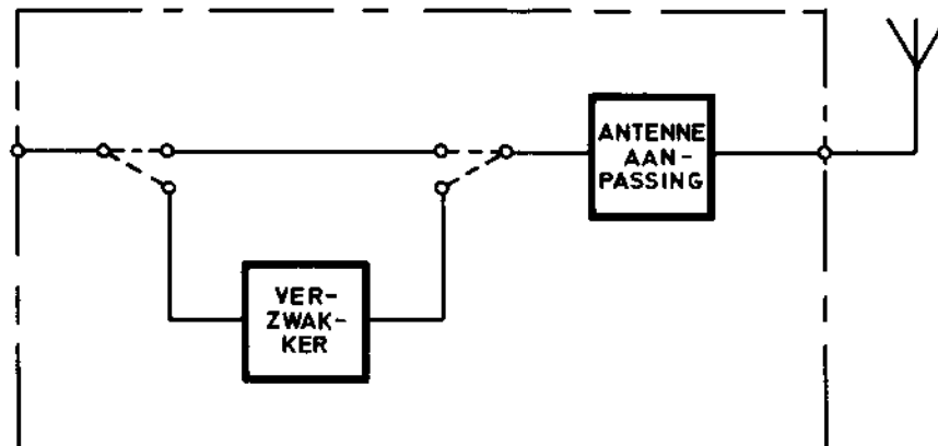
FIGUUR 7a BLOKSCHAMA, ANTENNE-AFSTEMEENHEID RF-3610
