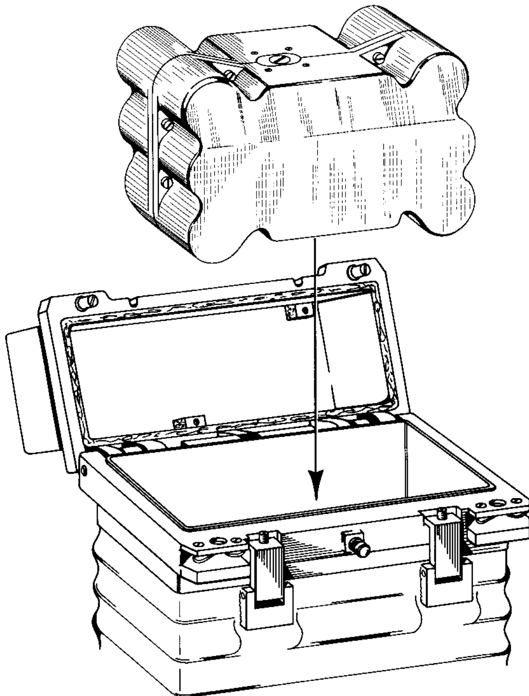
FIGUUR 57 HET VERVERGEN VAN DE ACCU IN DE BATTERIJHOUDER BX-3610
