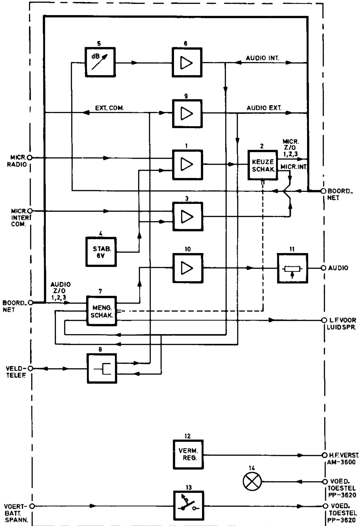
FIGUUR 8 BLOKSCHEMA, REGEL-EN INTERCOMMUNICATIE-EENHEID IC-3620
