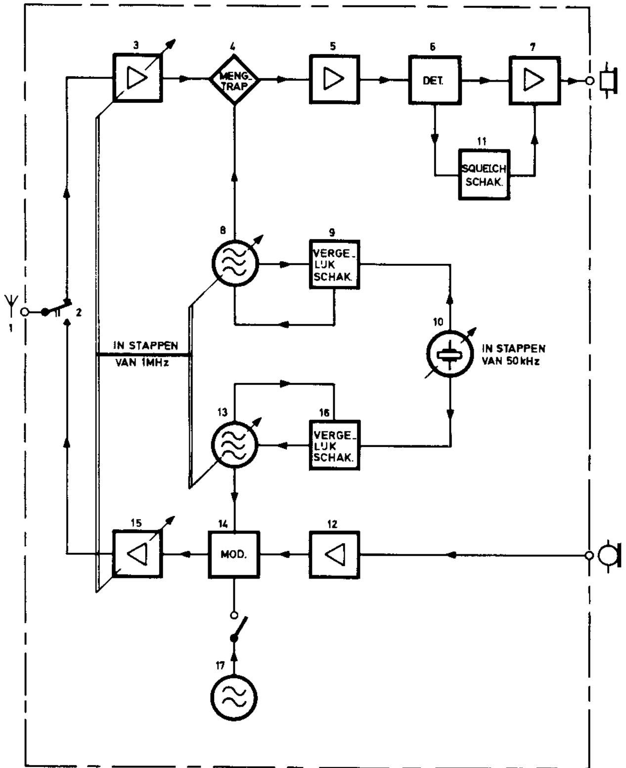
FIGUUR 1 ZENDER-ONTVANGER, RADIO
