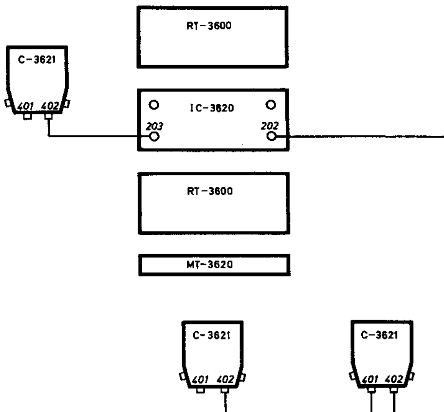
FIGUUR 42 VOORBEELDEN VOOR HET AANBRENGEN VAN EEN BOORDNET
